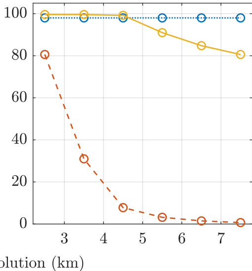
Mahalanobis
